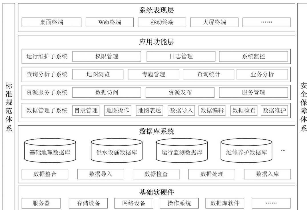
图 4.3.1 供水管网地理信息系统总体架构
